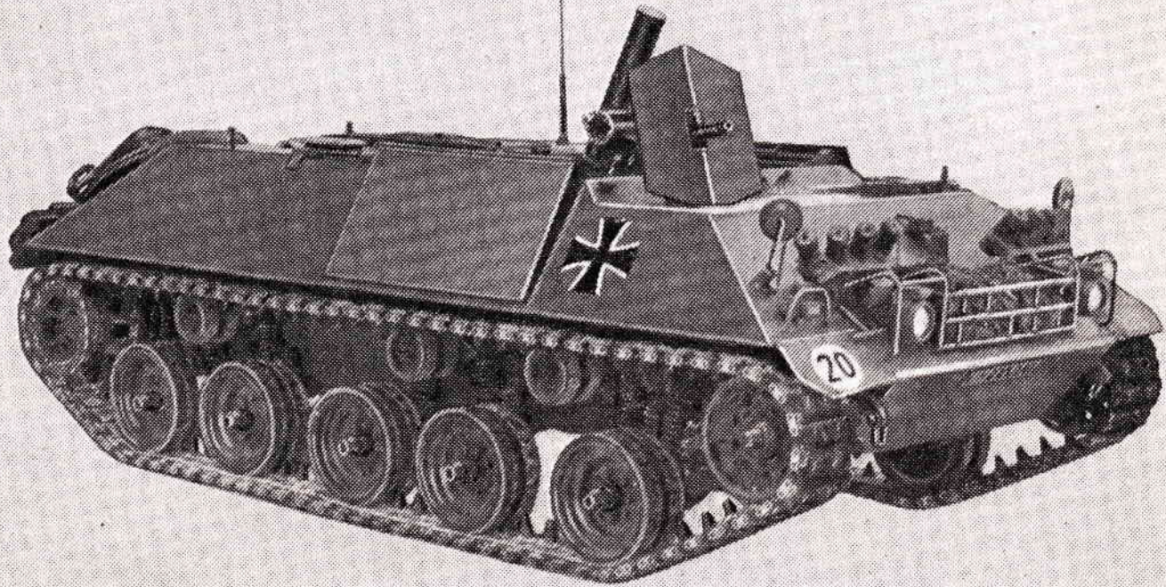
△ Mit MG und Schutzschild (auf allen anderen Abbildungen ist das MG abgenommen).
